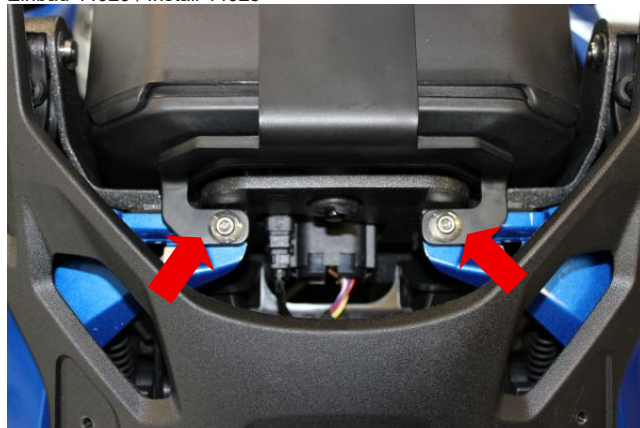
Einbau 44025 / Install 44025
